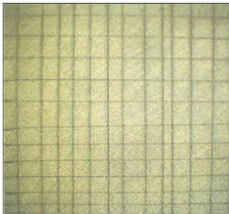
カッター刃による基盤目密着評価試験 100升試験にて剥離なし
