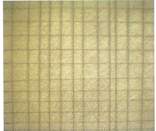
シリコンゴムへのクロスカット試験
