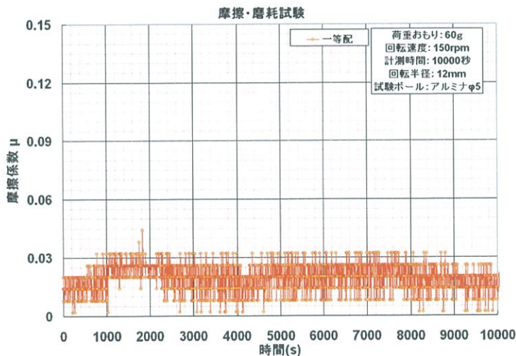
NBR(ニトリルゴム)への LF-DLC 摩擦・摩耗試験
